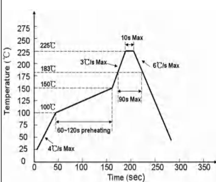
有铅焊接
